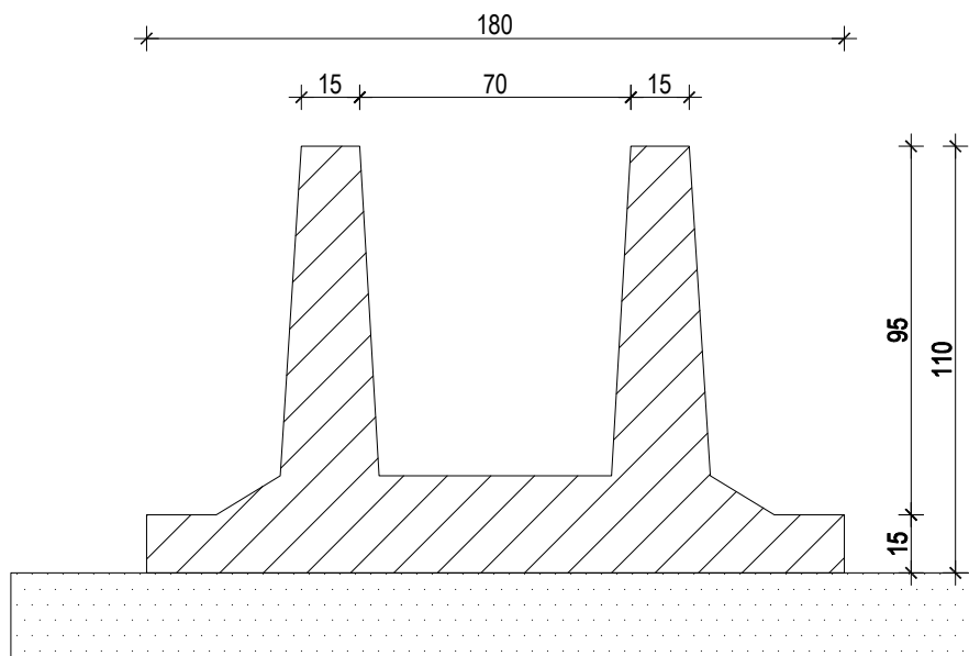
SEZIONE
